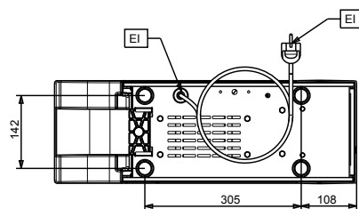
Boven aanzicht
